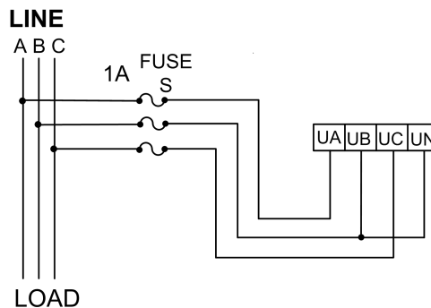
三相三线V型 (2LL)
